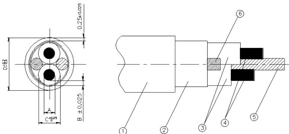
Рис. 2. Устройство нагревательного кабеля для матов Veria Quickmat (двухжильный нагревательный мат)
